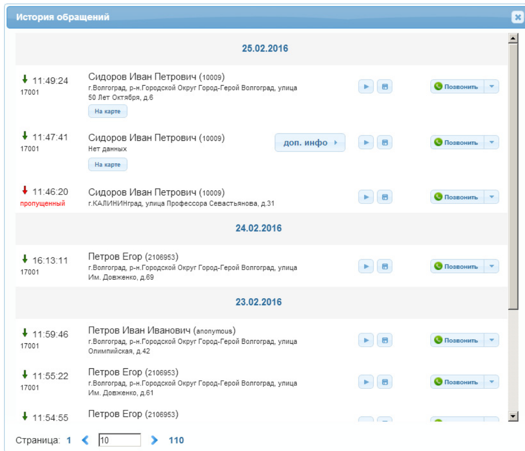
Рисунок 6-8: История обращений
